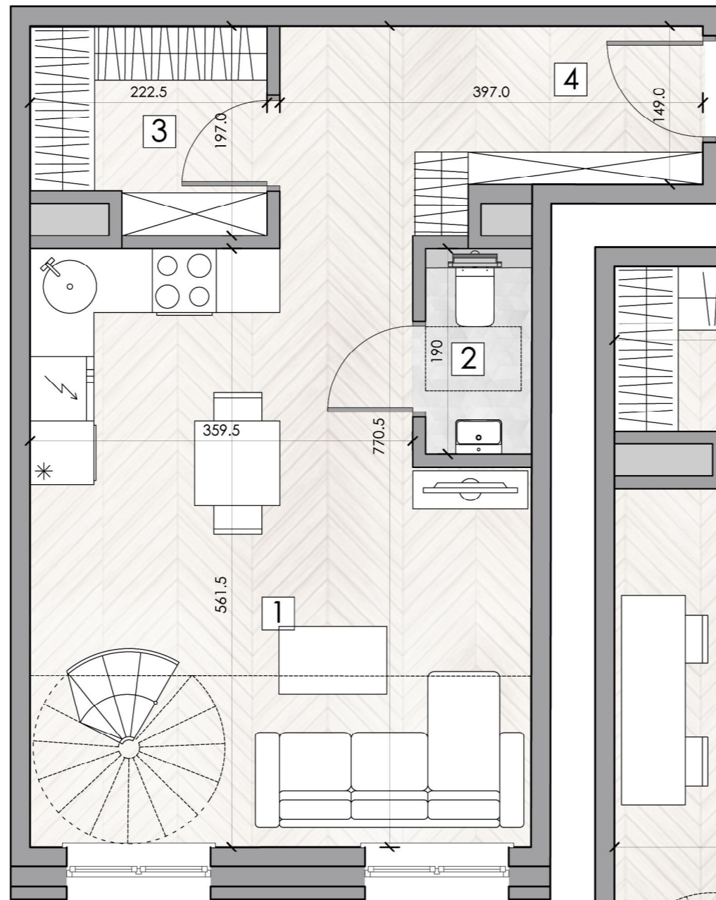
POZIOM +1
